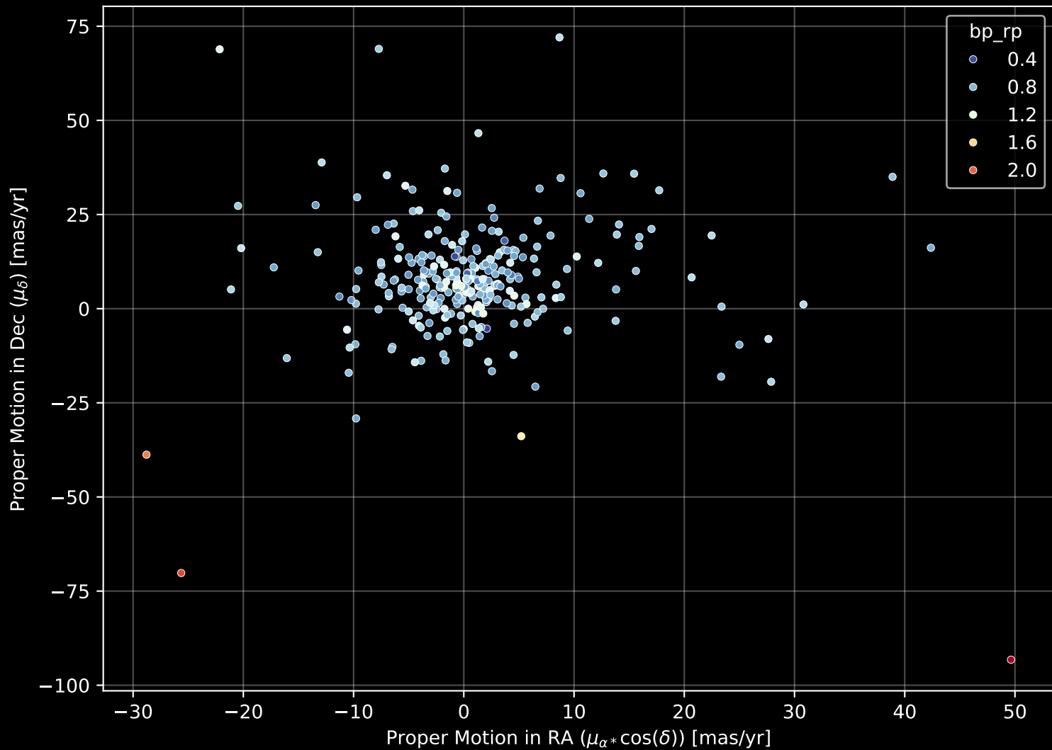
GALAH DR4 Field: [1079] Proper Motion Diagram (n= 295)
