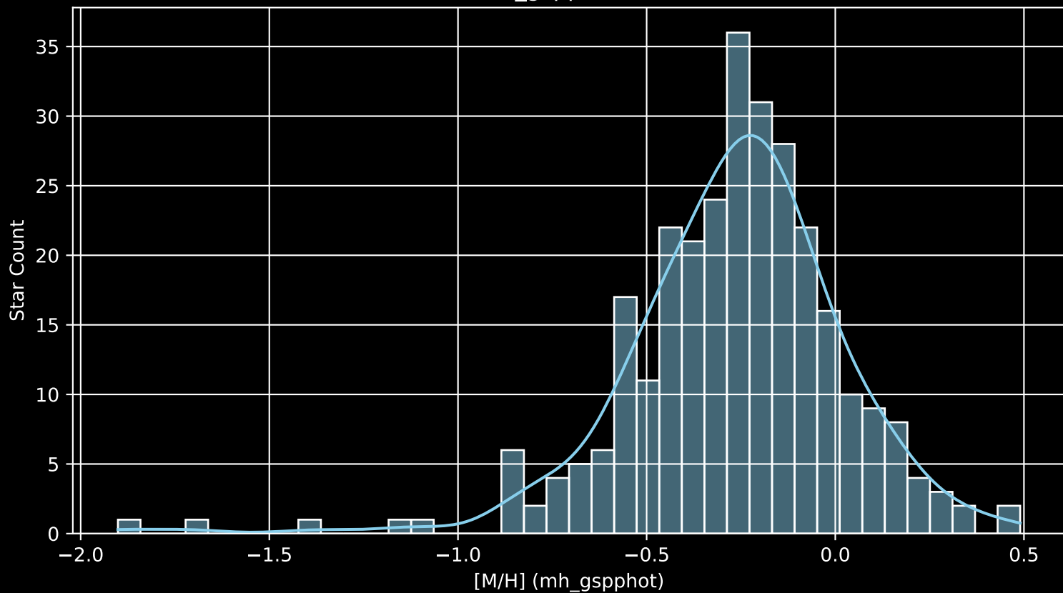
GALAH DR4 Field: [1079] [M/H] (mh_gspphot) (n= 294)
