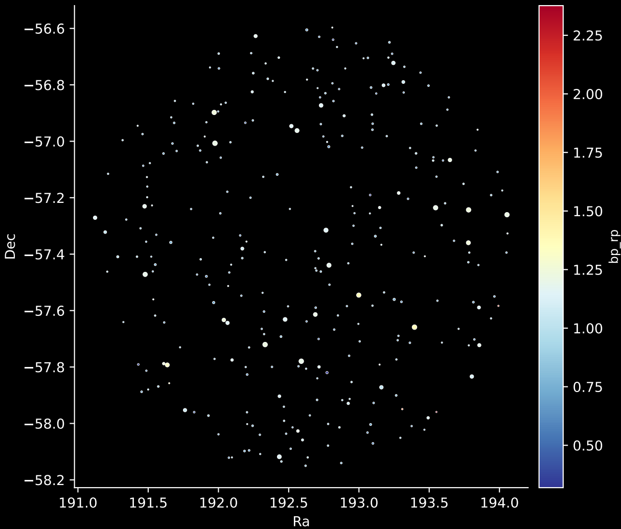
GALAH DR4 Field: [1079] Stars: 295
