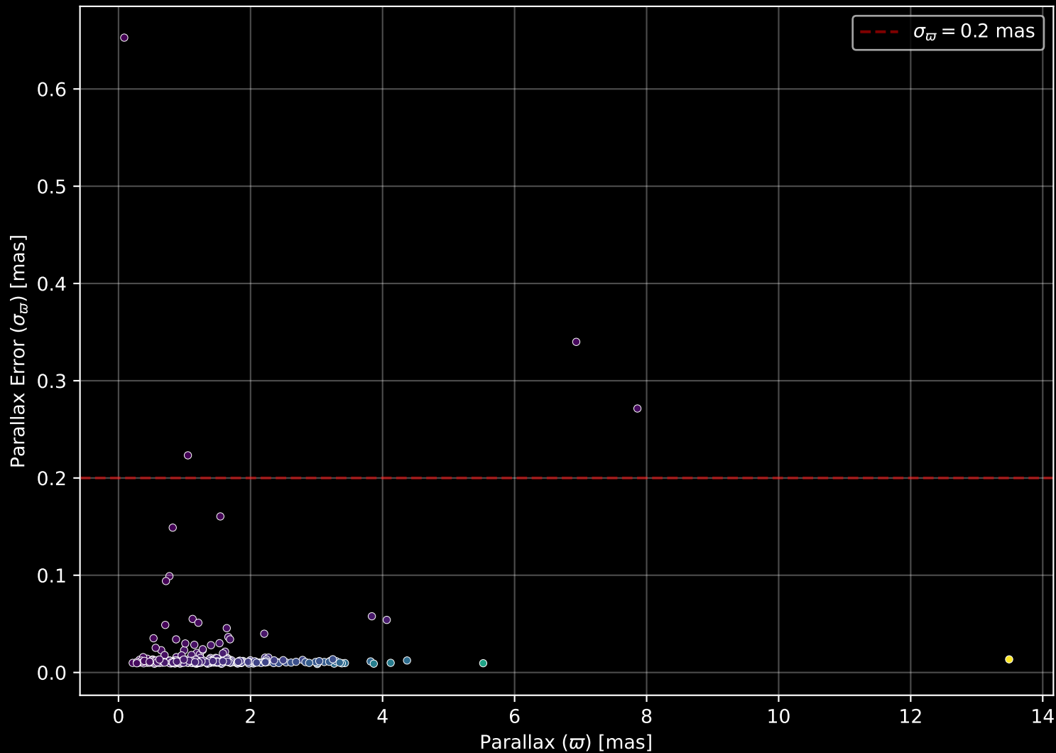
GALAH DR4 Field: [1079] Parallax Quality (n= 295)
