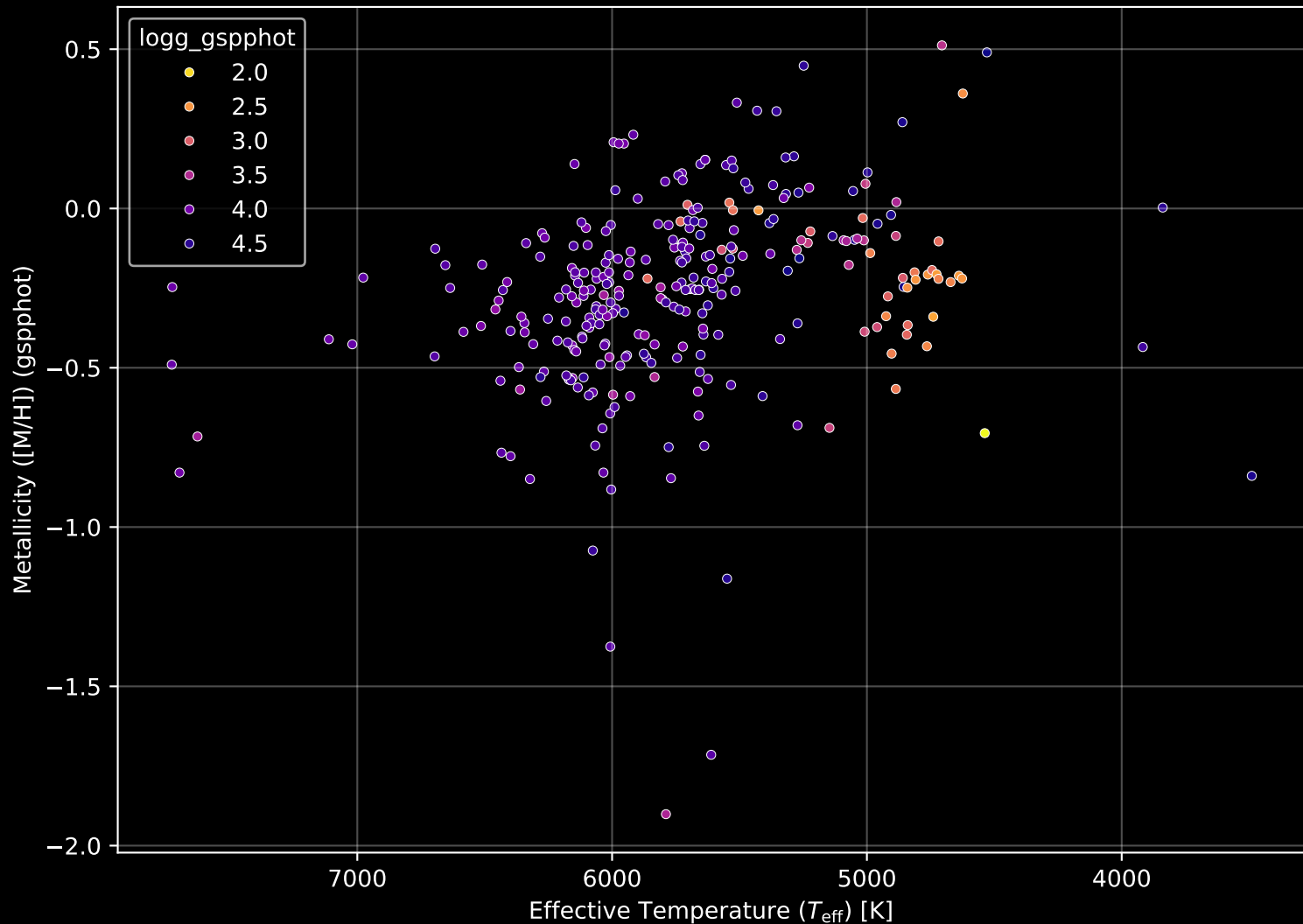
GALAH DR4 Field: [1079] Stellar Population Parameters (n= 295)
